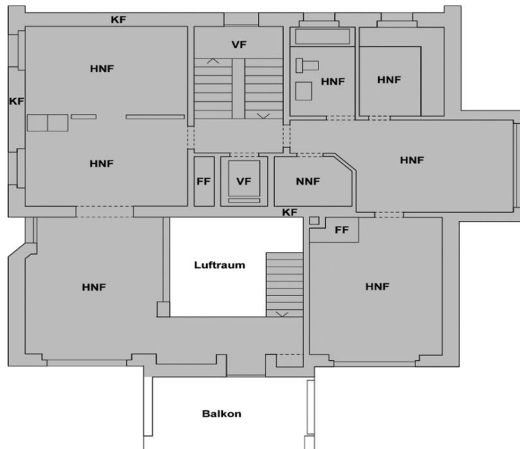
Grundriss 1. Obergeschoss:
